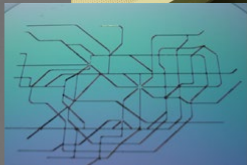
試作する東京地下鉄路線網マイクロ流路チップ。試作後、第6回で陽極接合。
